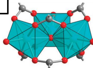
MIL-101(Cr)
