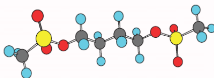
Busulfan
